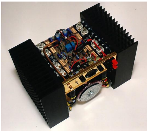
Open onderkant SOURCE mono eindversterker
