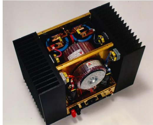
Open bovenkant SOURCE mono eindversterker
